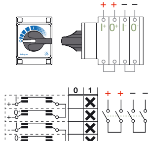
TFV1022 2 polos / 4 pisos 1 2 3 4 5 6 7 8 9 10 11 12 TFV1022
