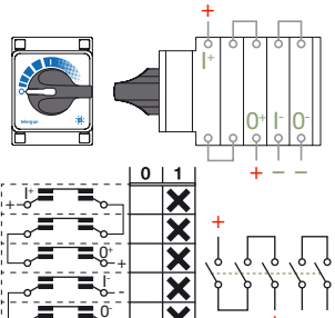
TFV1032 2 polos / 5 pisos 1 2 3 4 5 6 7 8 9 10 11 12 TFV1032
