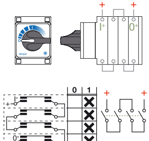
TFV1040 1 polo / 4 pisos 1 2 3 4 5 6 7 8 9 10 11 12 TFV1040
