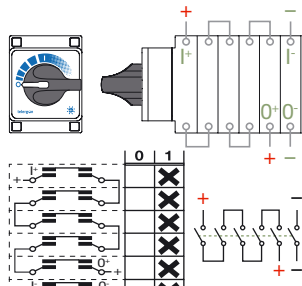
TFV1051 2 polos / 5 pisos 1 2 3 4 5 6 7 8 9 10 11 12 TFV1051
