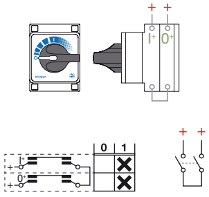
TFV0620 1 polo / 2 pisos 1 2 3 4 5 6 7 8 9 10 11 12 TFV0620
