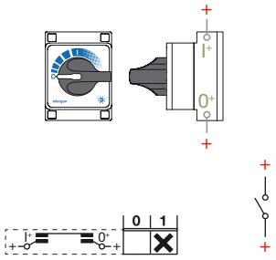
TFV0610 1 polo / 1 piso 1 2 3 4 5 6 7 8 9 10 11 12 TFV0610
