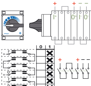
TFV1042 2 polos / 6 pisos 1 2 3 4 5 6 7 8 9 10 11 12 TFV1042
