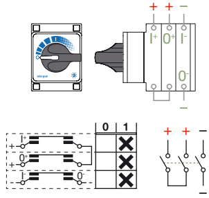
TFV1021 2 polos / 3 pisos 1 2 3 4 5 6 7 8 9 10 11 12 TFV1021
