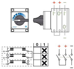
TFV0821 2 polos / 3 pisos 1 2 3 4 5 6 7 8 9 10 11 12 TFV0821
