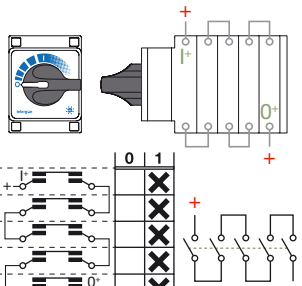
TFV1050 1 polo / 5 pisos 1 2 3 4 5 6 7 8 9 10 11 12 TFV1050
