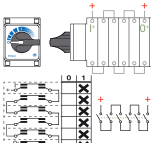
TFV1060 2 polos / 6 pisos 1 2 3 4 5 6 7 8 9 10 11 12 TFV1060
