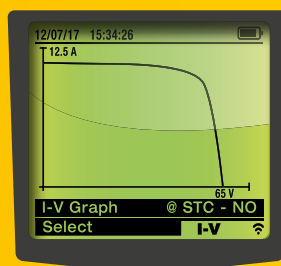
Resultado da curva I-V: OK
