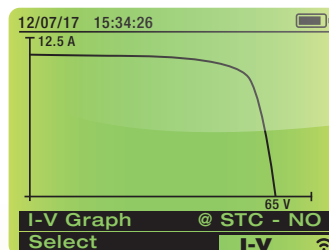
Resultado da curva I-V: OK
