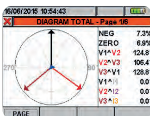
Diagrama do vetor de tensões e correntes
