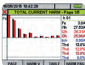
Exibição de harmônicos em tempo real
