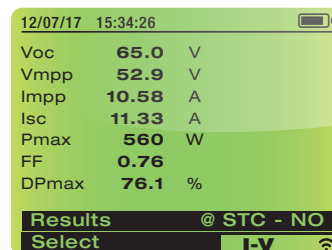
Detalhes da Curva I-V: OK
